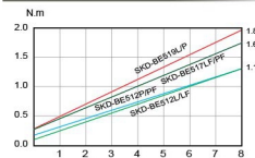
扭力曲線圖
